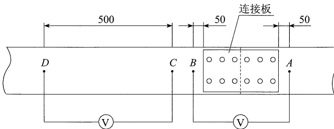
图 C.0.2 电气连续性试验布置
