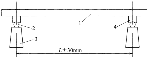
图 B.0.2 试验用支架示意
