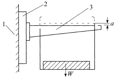
图 B.0.3-1 支架固定体和定位方式
