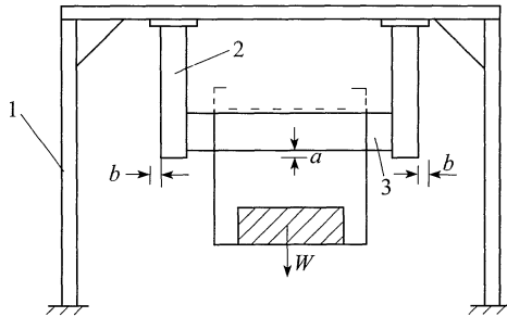
图 B.0.3-3 吊架固定体和定位方式
