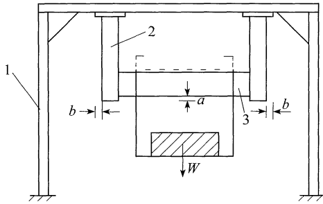
图 B.0.3-2 支架固定体和定位方式
